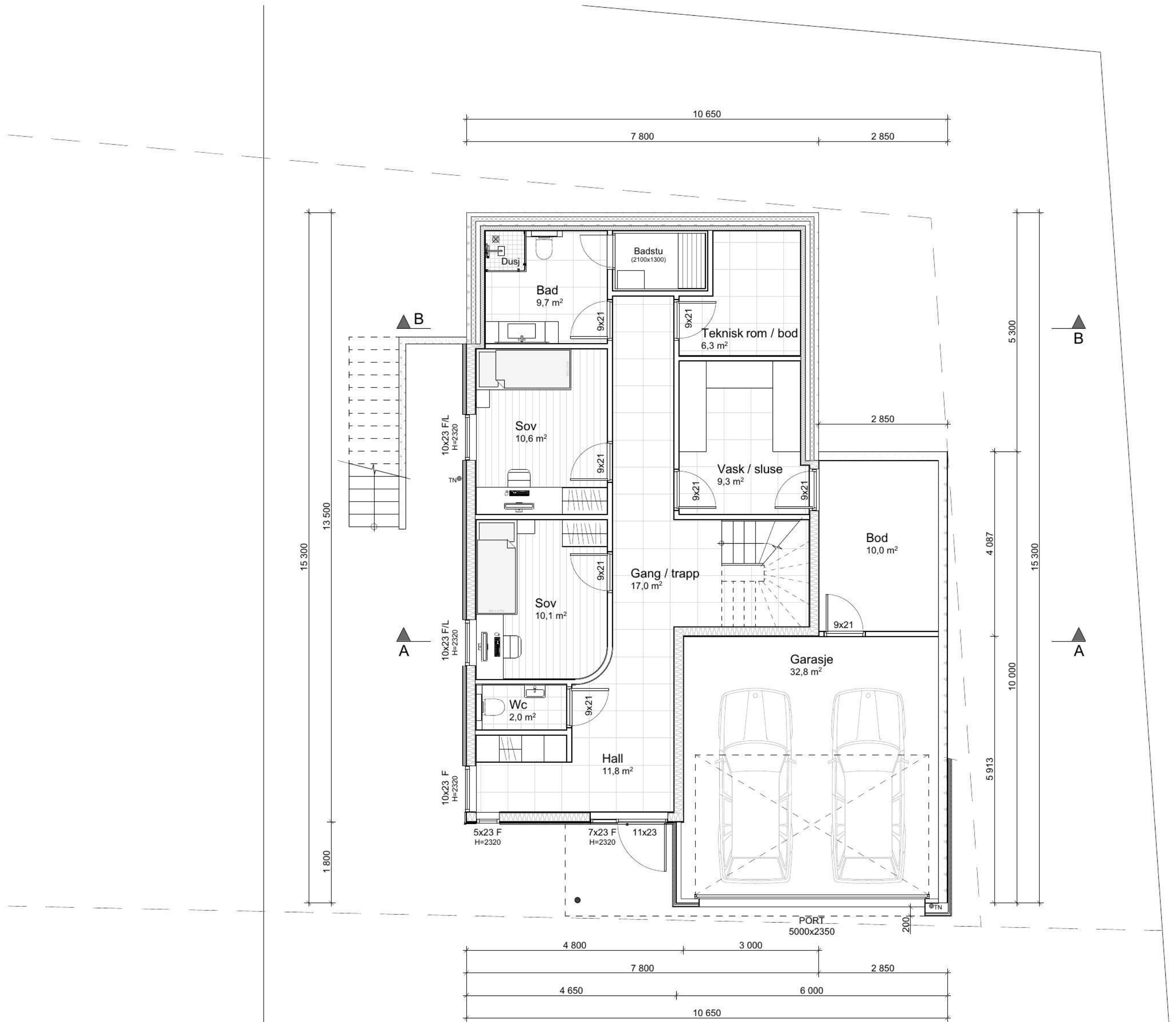
Plan 1.etasje BRA bolig A (inkl. garasje) 126,6 m²
